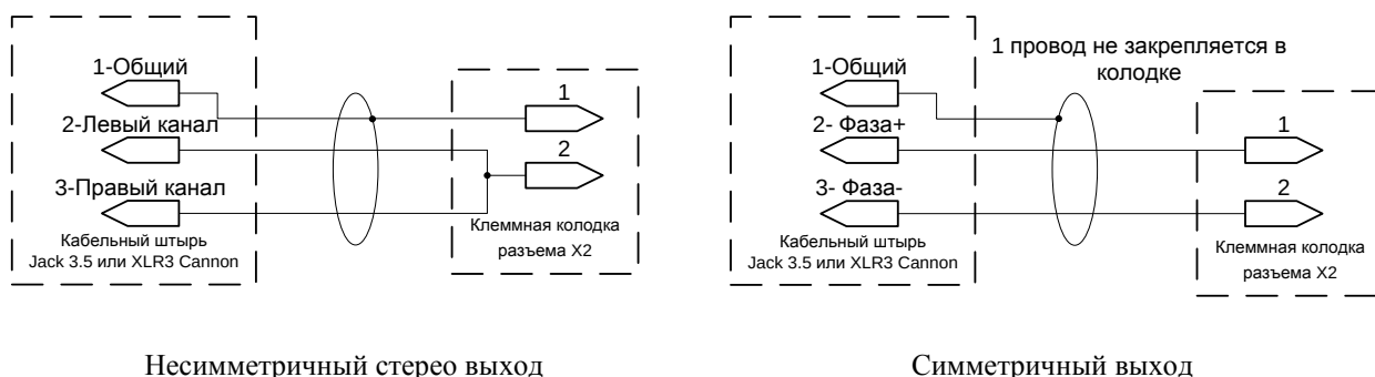
Рис. 6.1. Подключение шнуров Ш-3-1, Ш-4-1 к прибору.
