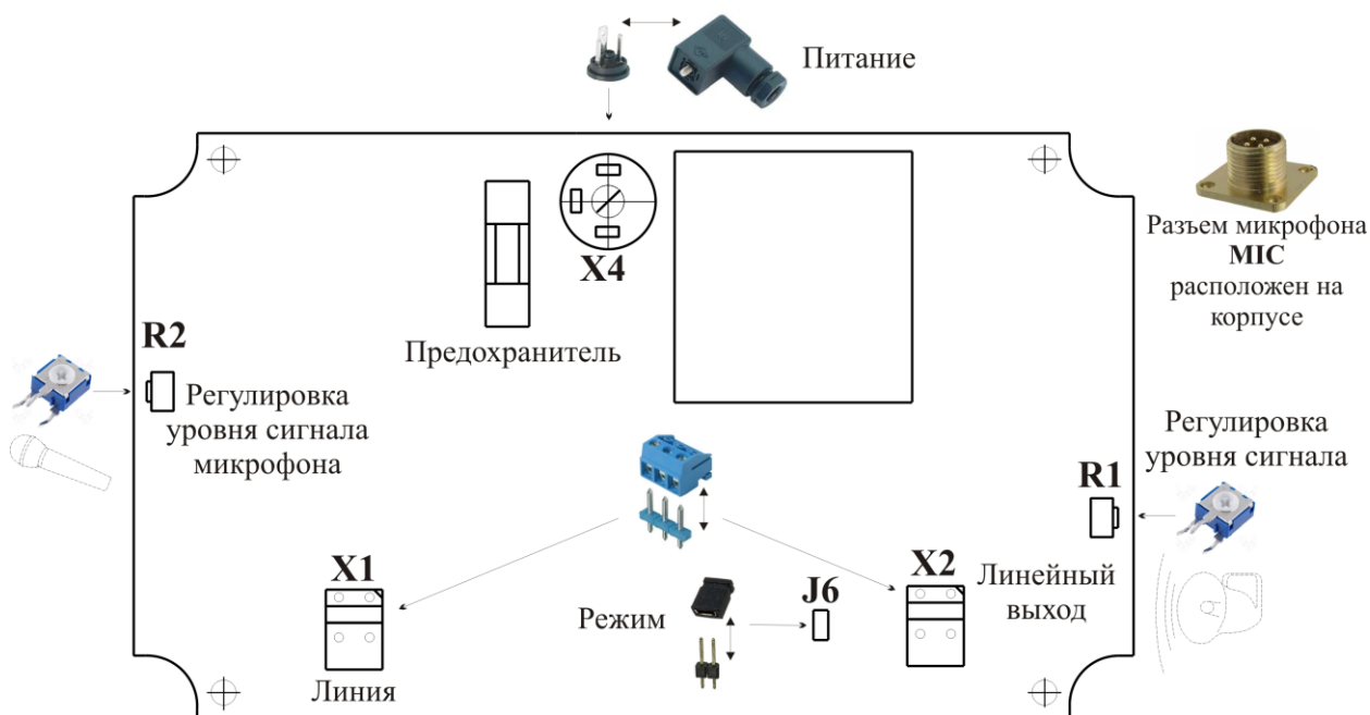
Рис.6 Размещение элементов на плате прибора
