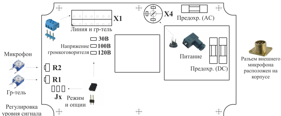
Рисунок 5 – Размещение элементов на плате прибора Тема-хх-А11.х2-xxx-х65
