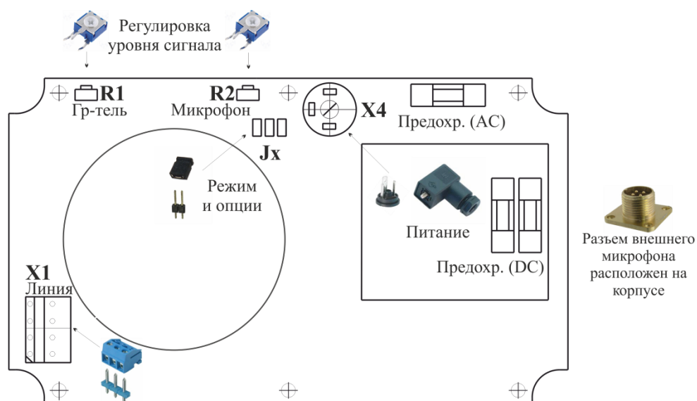
Рисунок 6 – Размещение элементов на плате прибора Тема-А12.х2-xxx-х65
