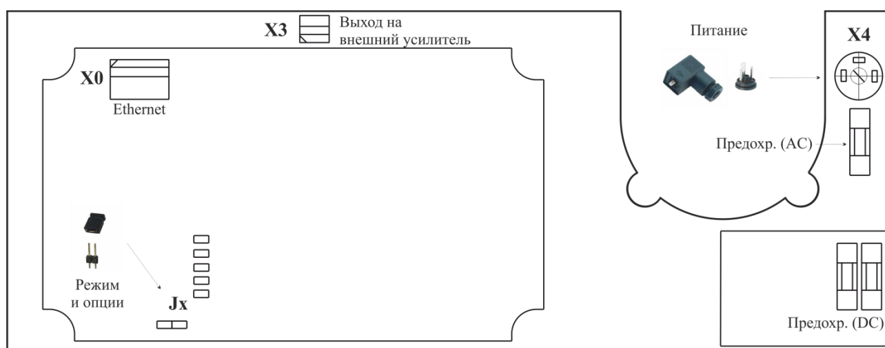
Рисунок 5 – Размещение элементов на нижней плате консоли Тема-АРК242.27-m51
