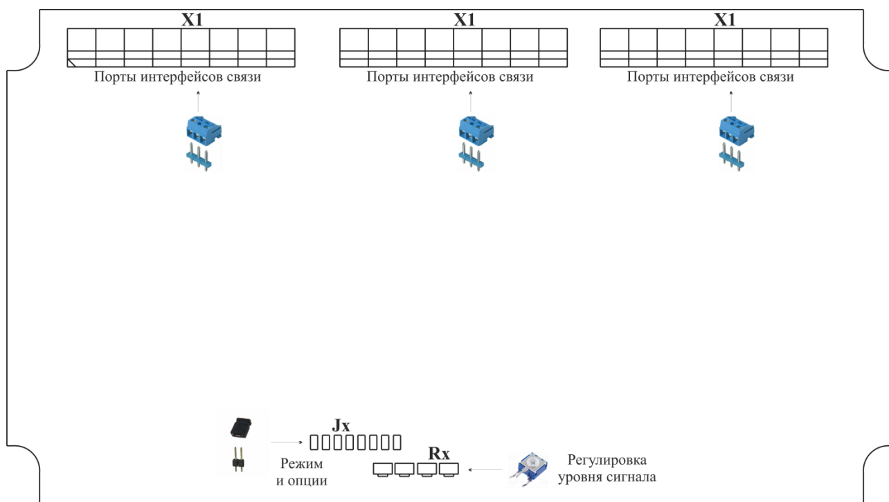
Рисунок 7 – Размещение элементов на верхней плате блока линий Tema-APM240.02-m65
