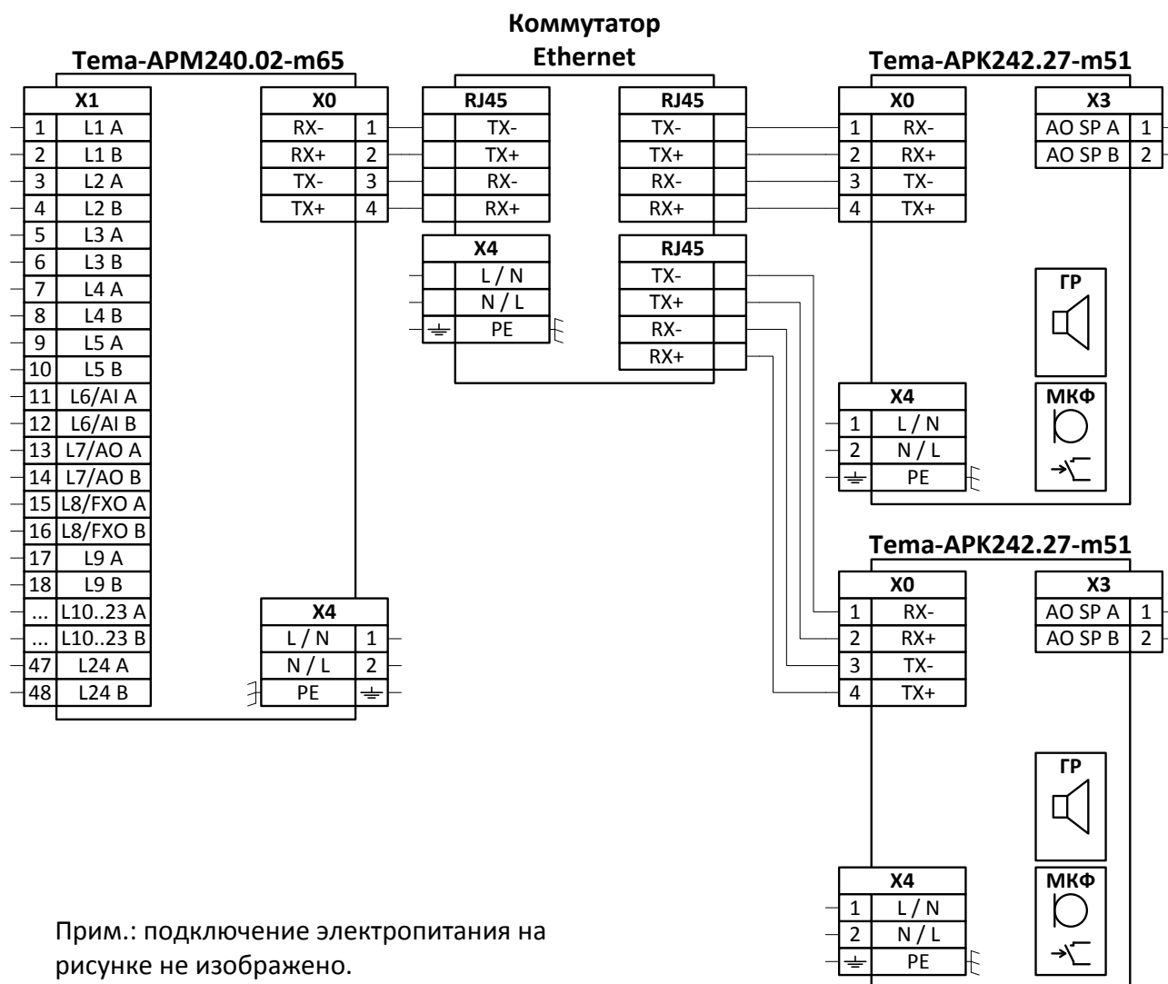
Рисунок 10 – Пример схемы подключения нескольких консолей к одному блоку линий
