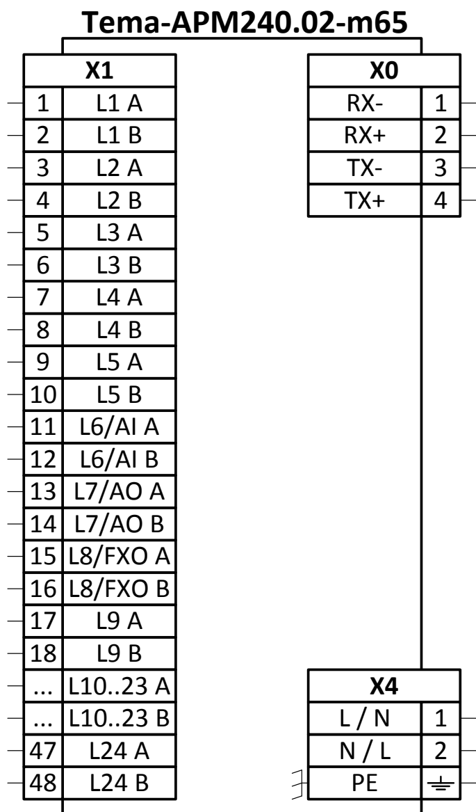
Рисунок 4 – Условное графическое обозначение блока линий Тема-APM240.02-xxx-m65
