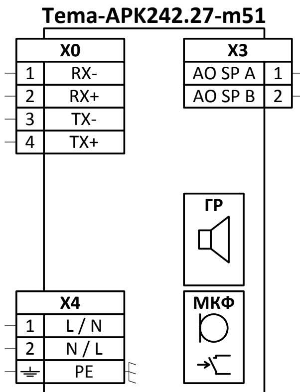
Рисунок 3 – Условное графическое обозначение консоли Тема-АРК242.27-xxx-m51
