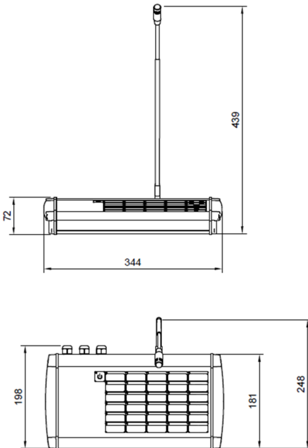
Рисунок А.2 – Габаритные размеры приборов Тема в настольном исполнении
