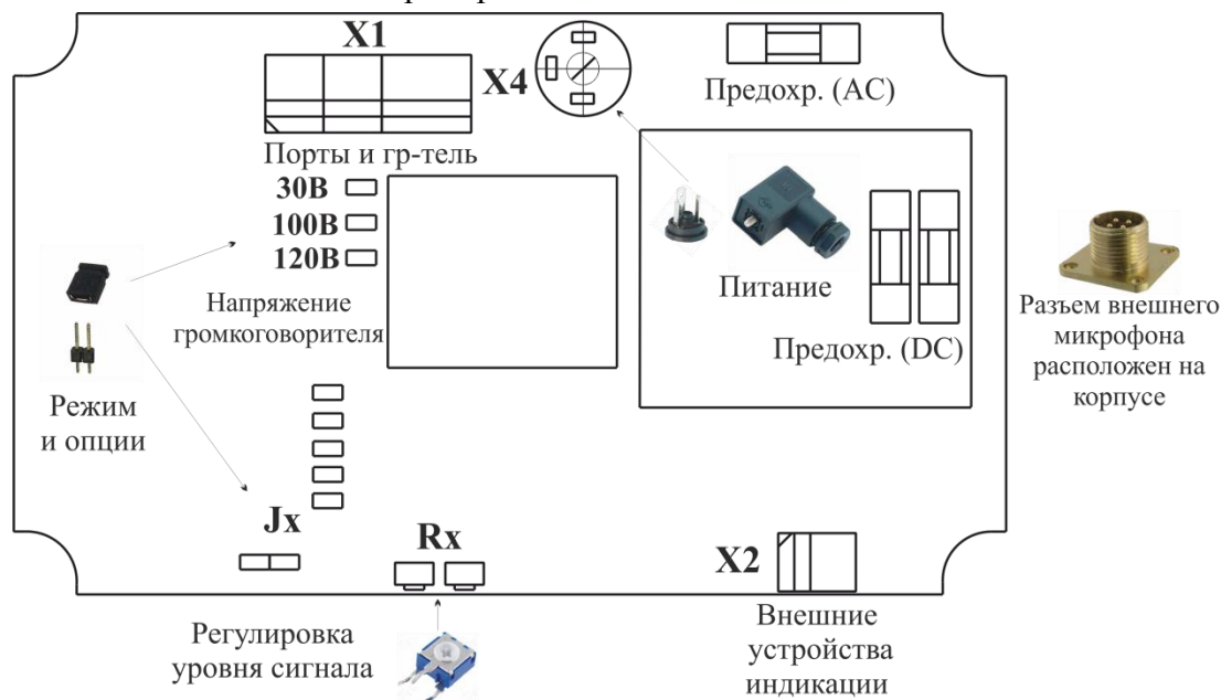
Рисунок 5 – Размещение элементов на плате прибора
