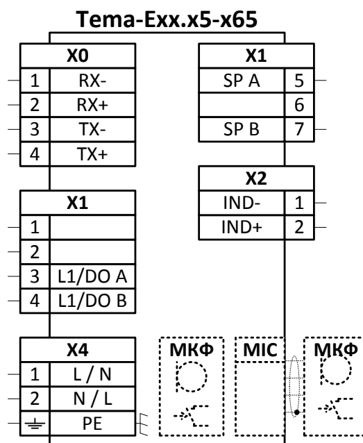
Рисунок 4 – Условное графическое обозначение прибора Тема-Ехх.х5-xxx-х65
