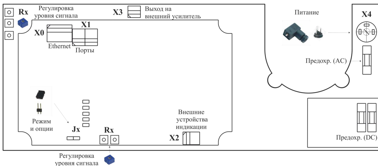
Рисунок 6 – Размещение элементов на плате прибора Тема-Мхх.х5-м51
