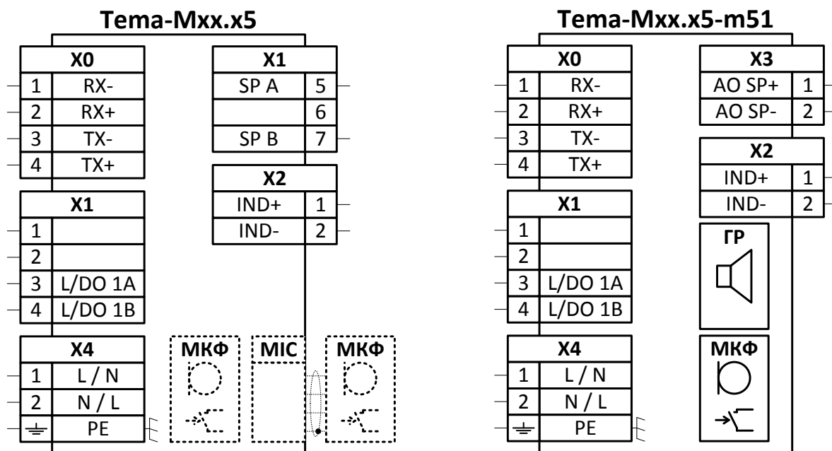
Рисунок 5 – Условное графическое обозначение прибора Тема-Мхх.х5
