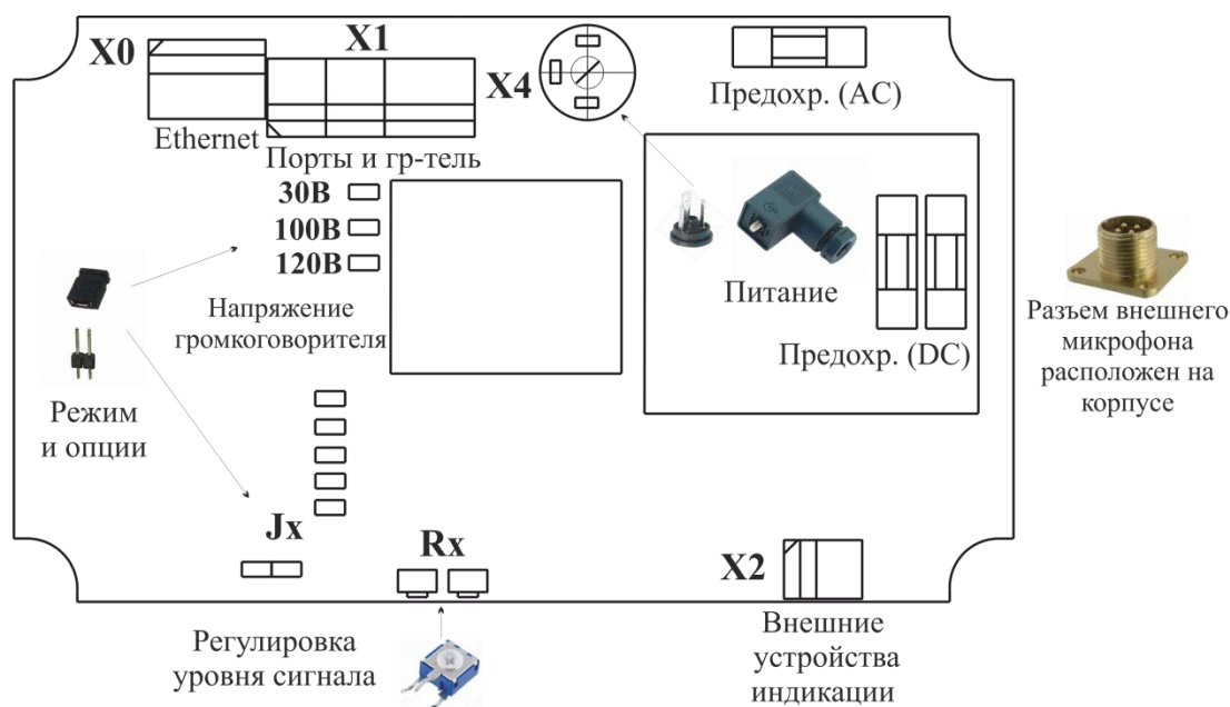
Рисунок 7 – Размещение элементов на плате прибора Тема-Мхх.х5-х65
