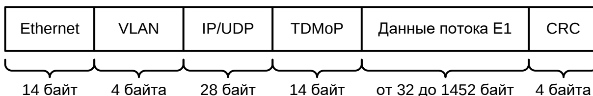
Рис. 5 Формат пакета с данными потока E1
